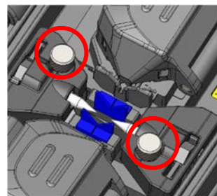
电极棒的固定板螺丝
