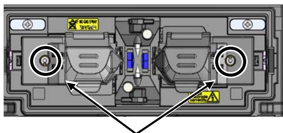
涂覆层裸光纤夹具固定螺丝
