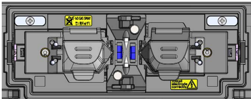
使用 60mm 热缩套管
